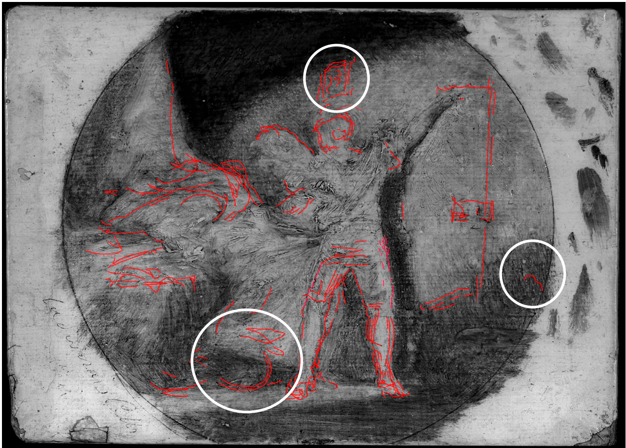
Le Verrou ovale, relevé du dessin sous-jacent grâce à la réflectographie infrarouge (Art in Lab, Paris).
